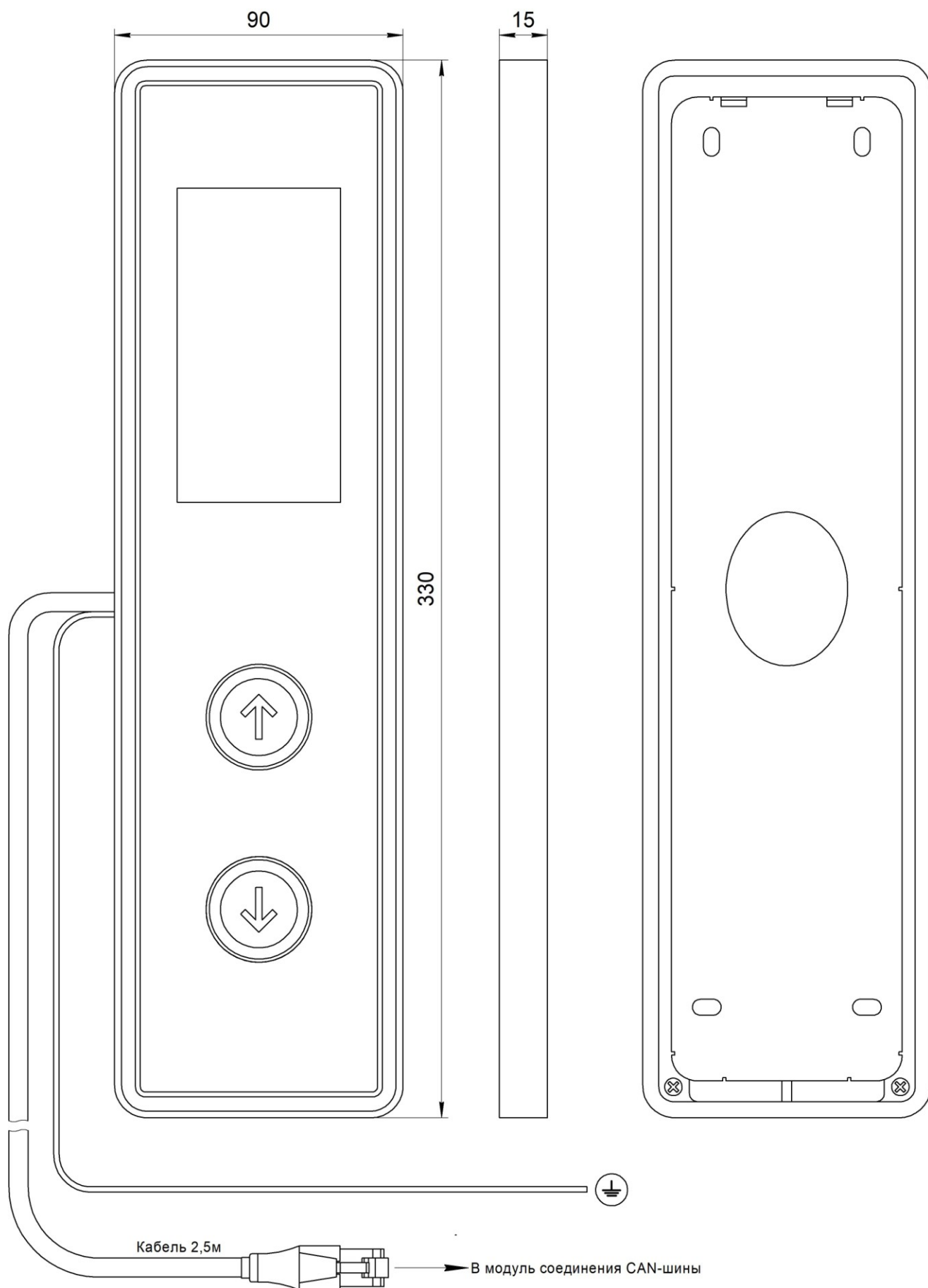
Рис.1 Внешний вид, габаритные и установочные размеры Вызывного поста ОБСИДИАН (жгут RJ45) НШЕК.468381.228
